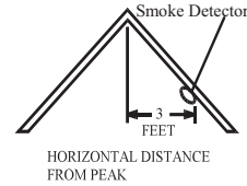
Рисунок 5: РЕКОМЕНДУЕМОЕ РАСПОЛОЖЕНИЕ ДАТЧИКОВ ДЫМА В ПОМЕЩЕНИЯХ С ОСТРОКОНЕЧНЫМИ ПОТОЛКАМИ
