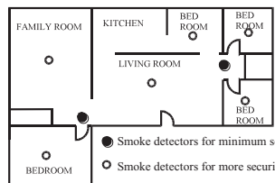
Рисунок 2: МЕСТОПОЛОЖЕНИЕ ДЛЯ УСТАНОВКИ ДАТЧИКА ДЫМА В КВАРТИРЕ С БОЛЕЕ ЧЕМ ОДНОЙ СПАЛЬНОЙ ЗОНОЙ
